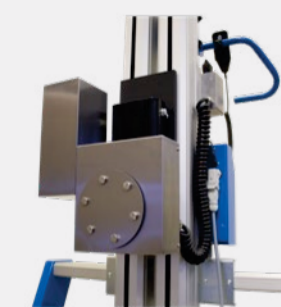
Turning Module
